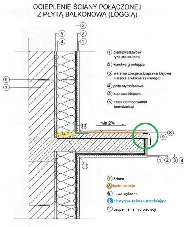
ELASTYCZNA TAŚMA USZCZELNIAJĄCA W NAROZU ZEWNĘTRZNYM
